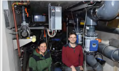
Requenzgeregelte Hocheffizienz- pumpen Freibadverein Lichtenau
